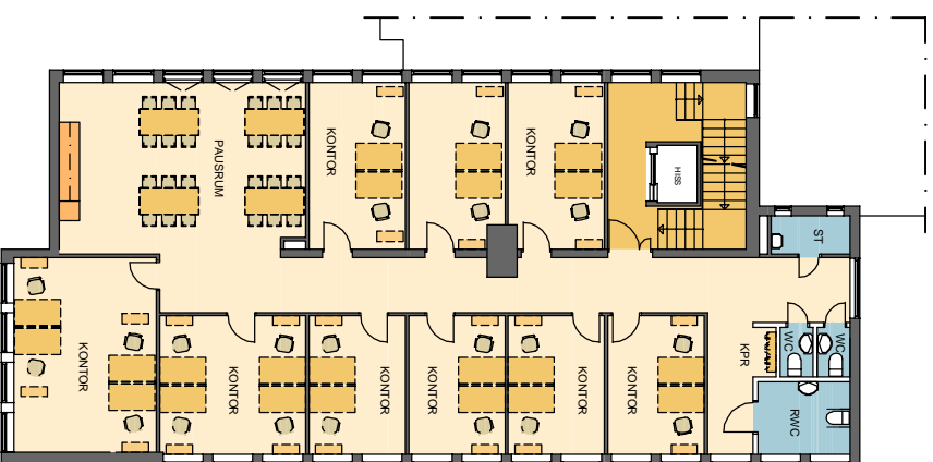
FÖRSLAG UTFÖRANDE PLAN 3-4 LOKAL 240 m 2
