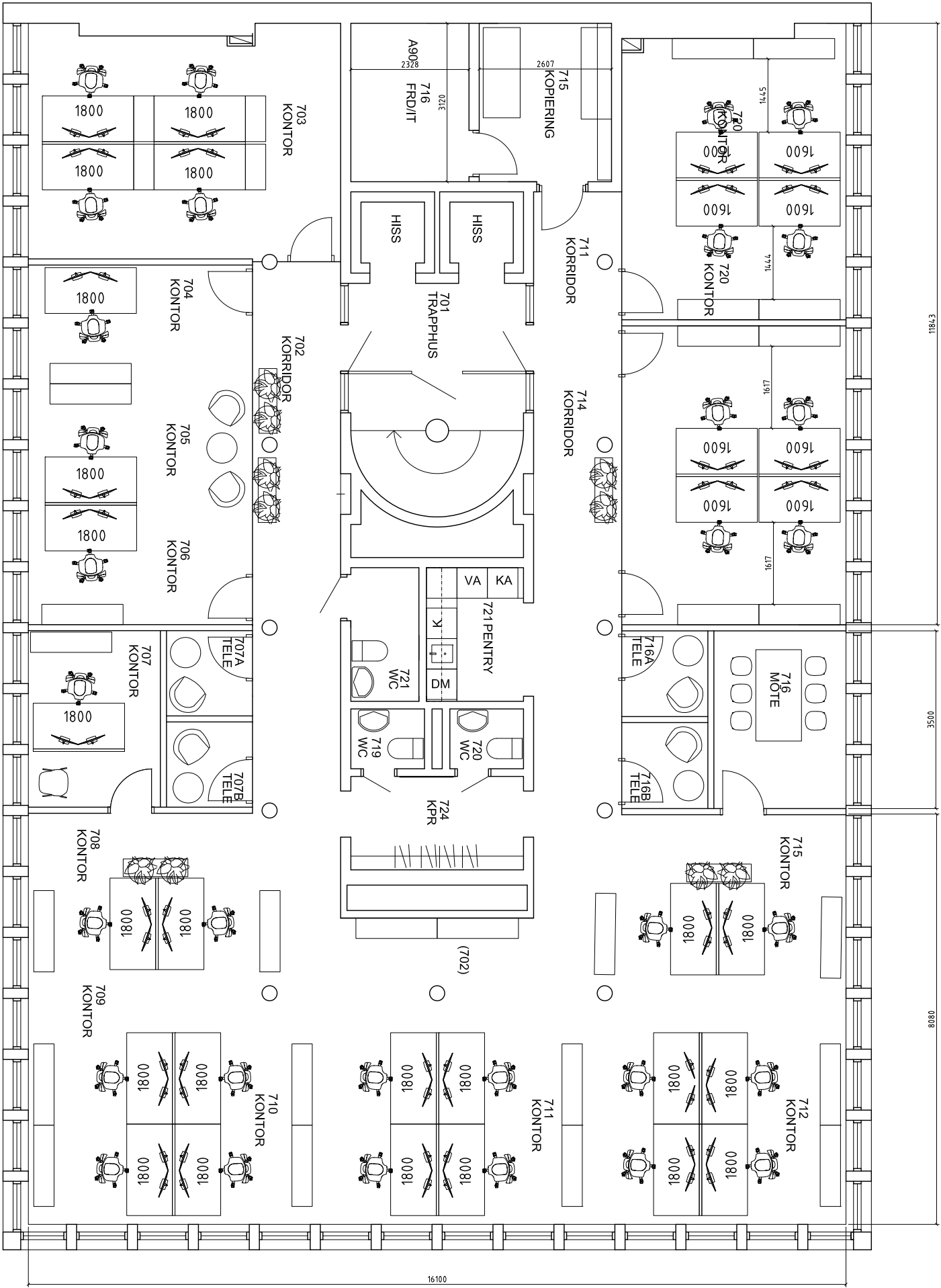
PLAN 7 MÖBLERINGSFÖRSLAG
