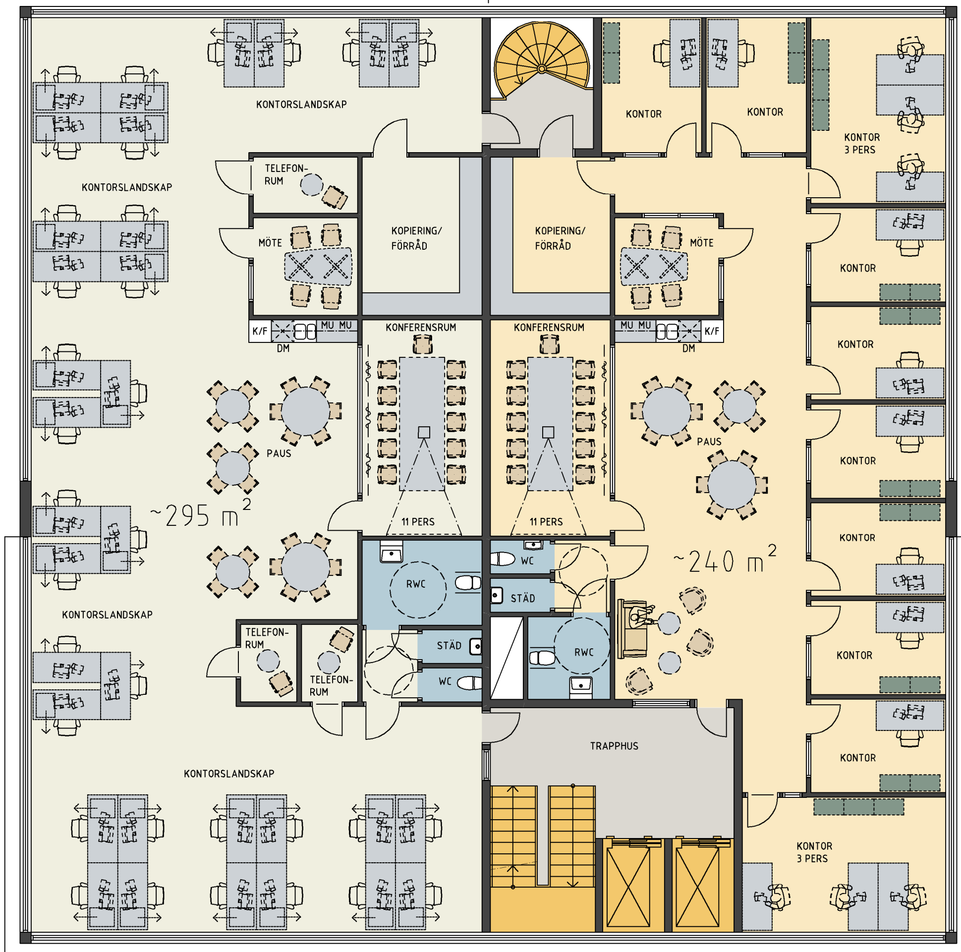
NYBYGGNAD PLAN, VÅNING 2 TR - 6 TR 1:100
